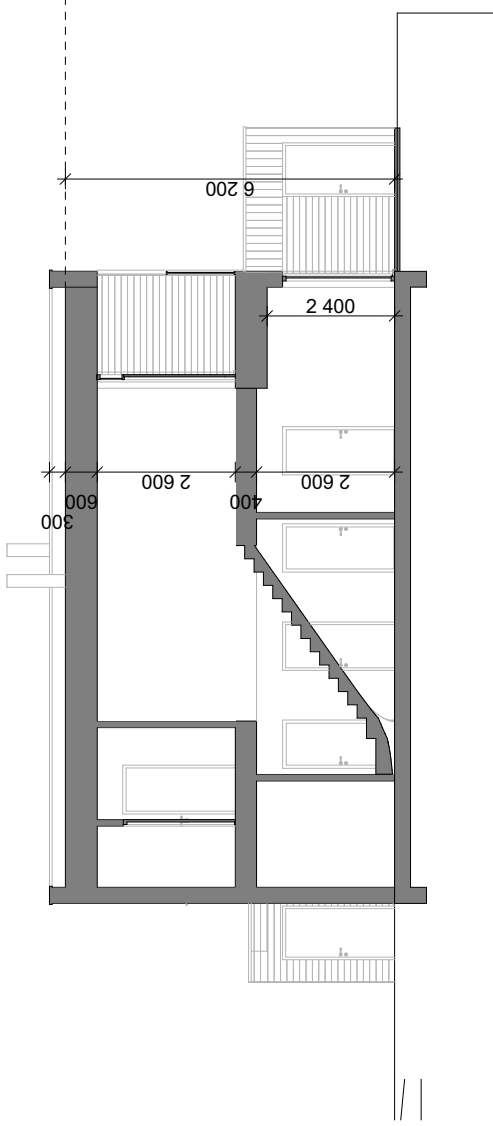
SNITT B - REKKEHUS B6
